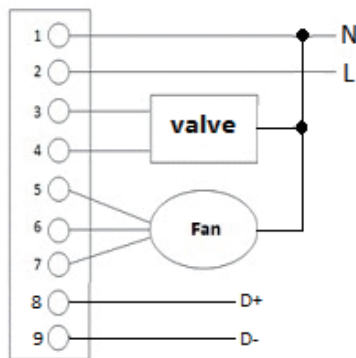
Fig. 3. Honeywell VC6013/VN6013 Wiring
