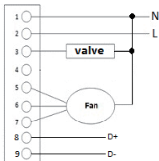
Fig. 2. Honeywell VC4013/VN4013/VS4016 Wiring
