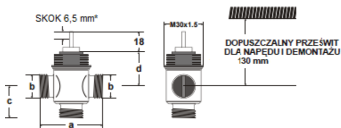
Rys. 6. Zawory 3-drogowe, wymiary (mm)
