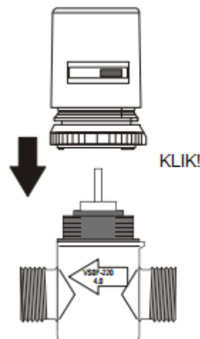
Rys. 4. Wbudowany zatrask
