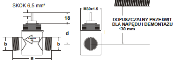
Rys. 5. Wymiary zaworów 2-drogowych (mm)
