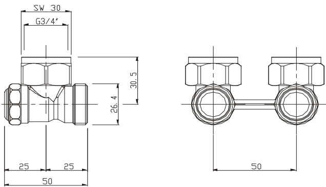
Rys. 1. Verafix-VK kątowy dla instalacji 2-rurowych
