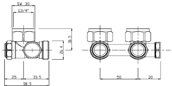
Rys. 2. Verafix-VK kątowy dla instalacji 1-rurowych
