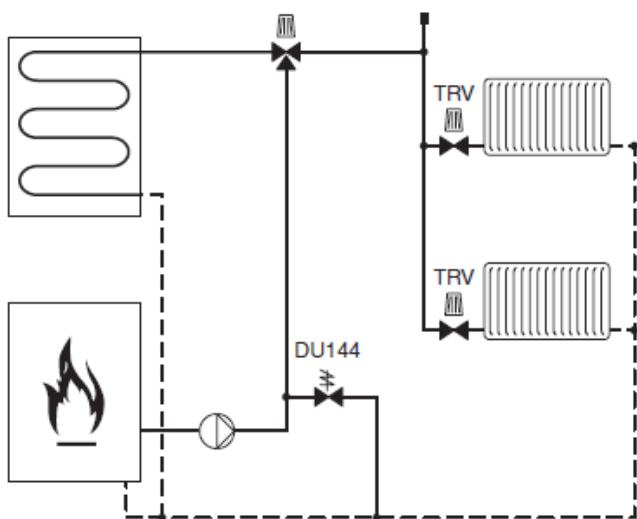
Rys. 4. DU144 w systemie z zasobnikiem
