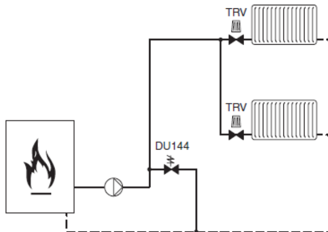
Rys. 5. DU144 w systemie z kotłem
