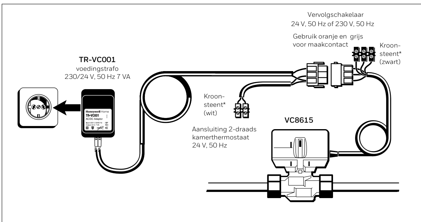
Fig. 5 Elektrische aansluiting VC8615
