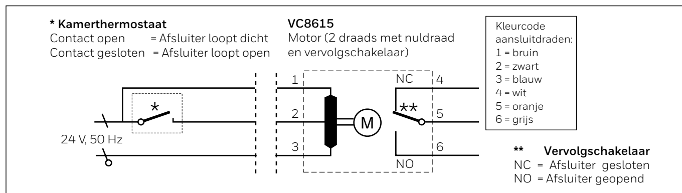
Fig. 4 Principeschema VC8615
