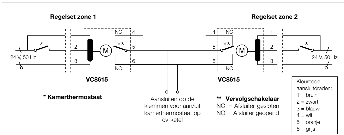
Fig. 7 Principe aansluitschema zoneregeling met 2 zones en cv-ketel
