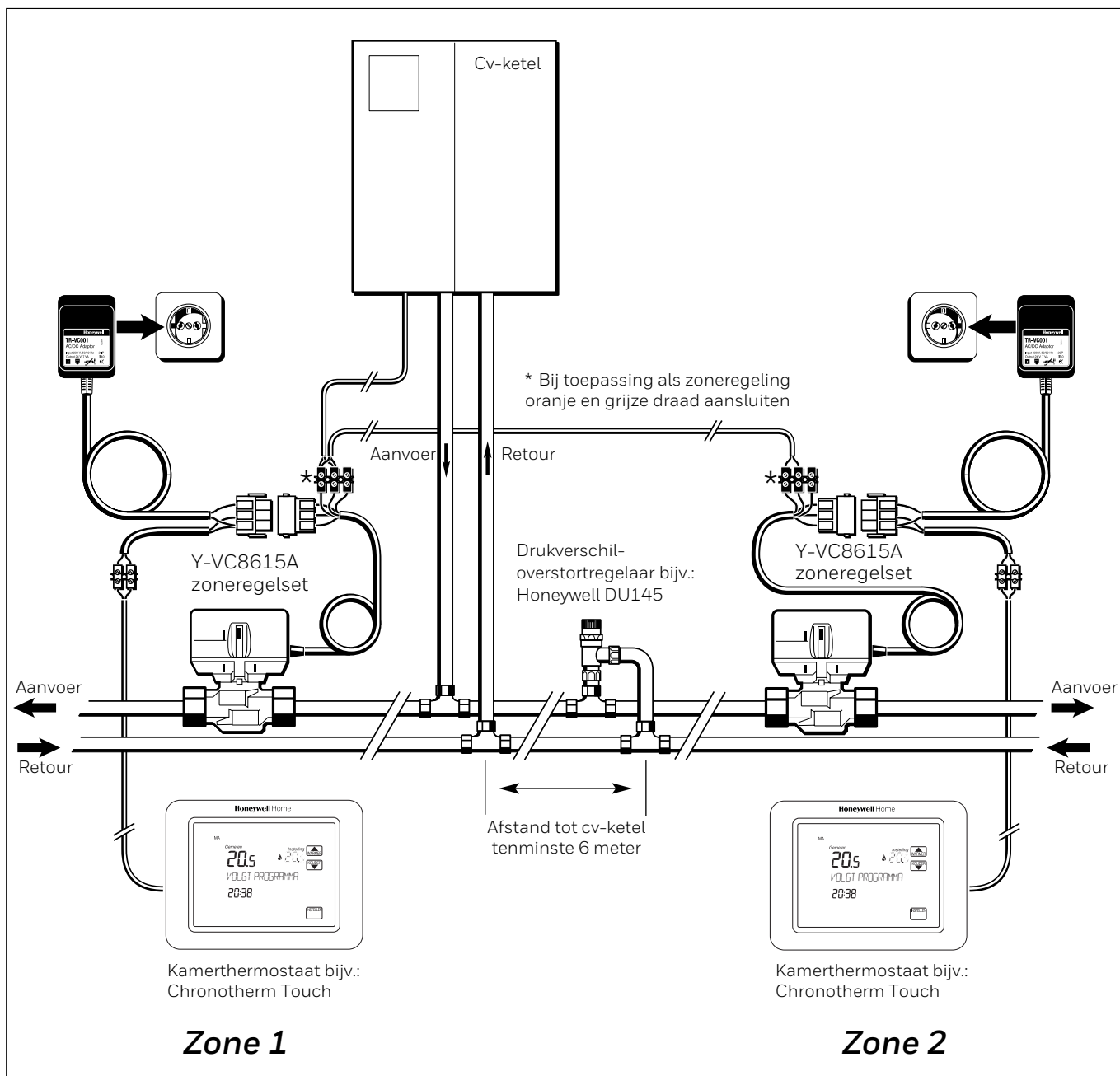
Fig. 9 Overzichtscha zoneregeling met 2 zones
