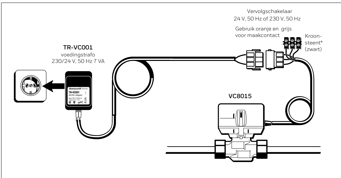
Fig. 5 Elektrische aansluiting VC8015
