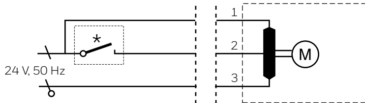
Fig. 4 Principeschema VC8015
