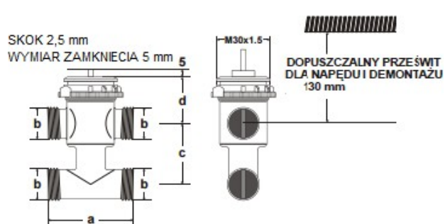
Rys. 10. Wymiary zaworów 3-drogowych z obejściem (mm)
