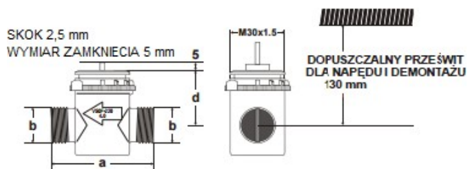
Rys. 8. Wymiary zaworów 2-drogowych (mm)
