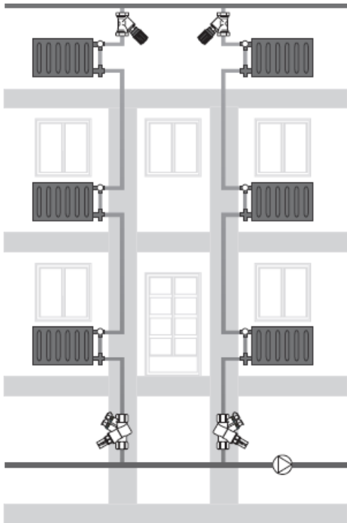
Rys. 2. Instalacja 1-rurowa
