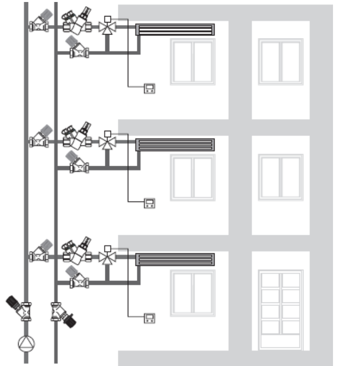
Rys. 3. Klimakonwektory z bypassem
