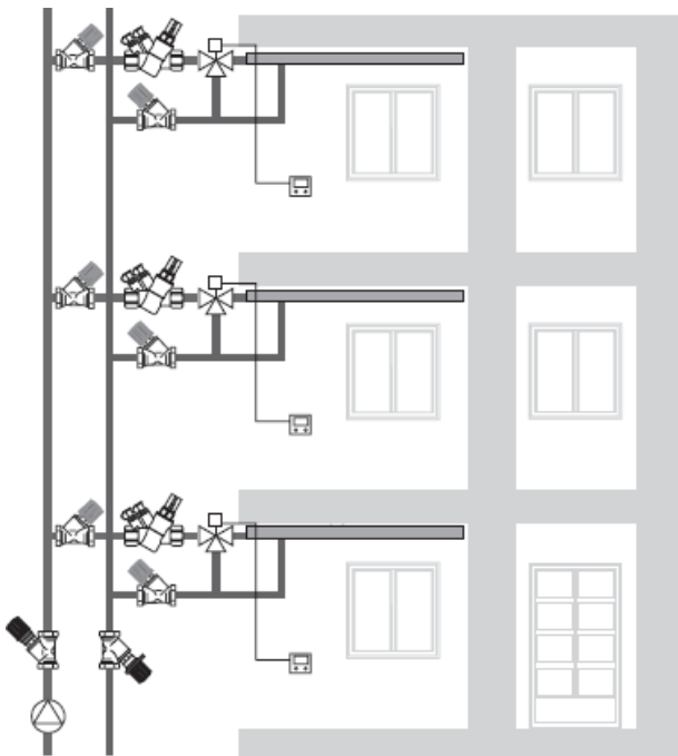
Rys. 4. Stropy chłodzące z bypassem
