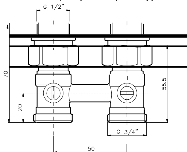
Rys. 4. Zawór Verafix-VKE prosty z płaską uszczelką i redukcją 3/4\"/>
