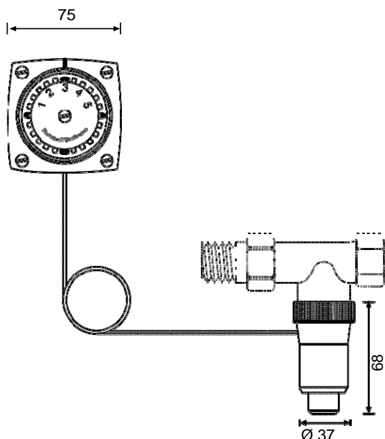
Fig. 1. Dimensioni T100MZ
