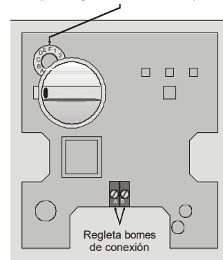
Fig. 2. SDW 10 (con tapa frontal quitada)
