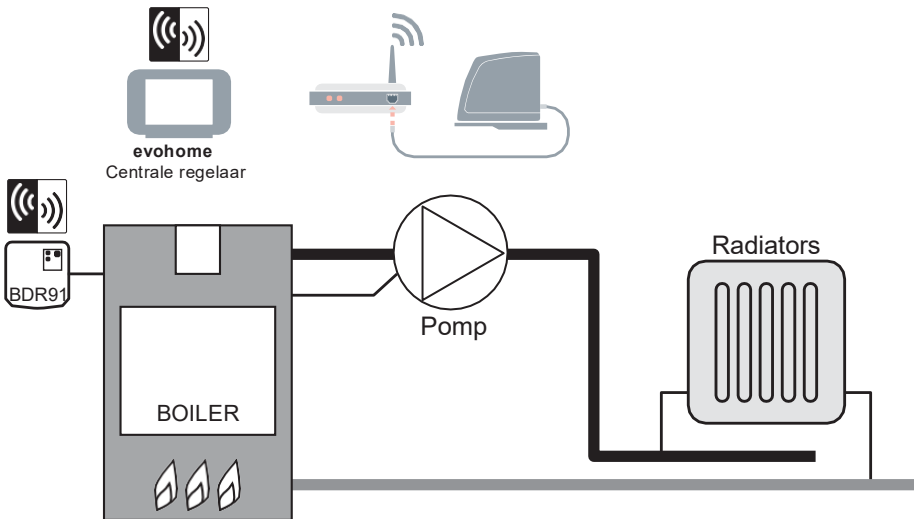
Afbeelding 1 Enkel zonesysteem
