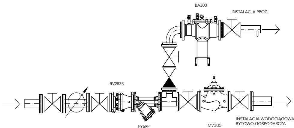
Rys. 2 Przykładowe zastosowanie zaworu elektromagnetycznego MV300
