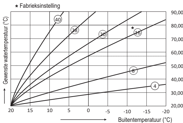
Stooklijn bij temperatuurstelling van 20 °C.
