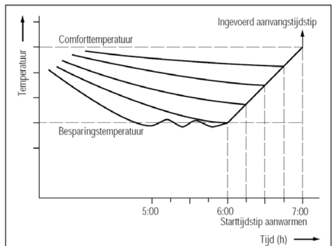
Figuur 4: Bepalen starttijd aanwarmen
