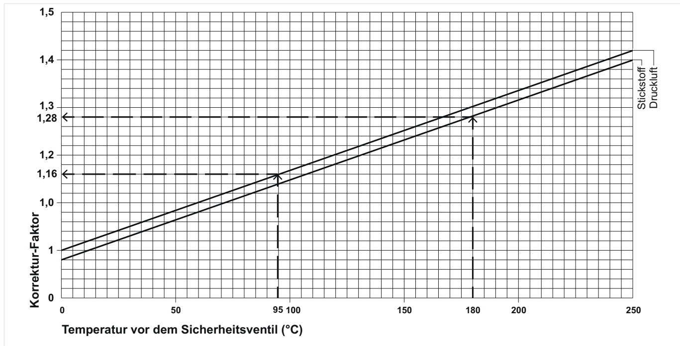
Abb. 2 Korrekturfaktor in Abhängigkeit von der Temperatur
